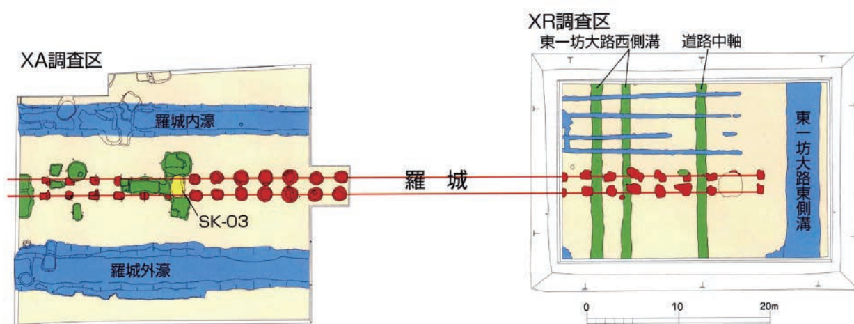
図2 2005年調査羅城遺構（現地説明会資料より一部改変。縮尺任意）
